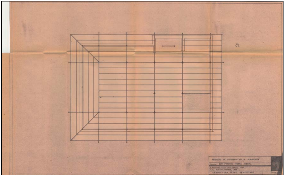
PLANO 04: PLANTA DE FORJADO DE TECHO DE SEMISÓTANO. E 1/50
