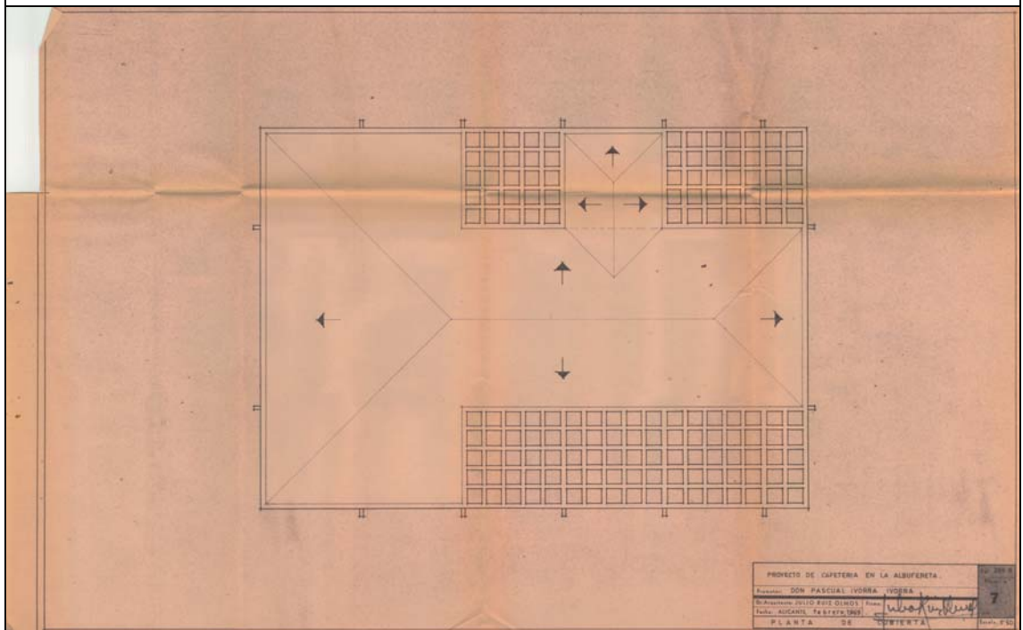
PLANO 07 PLANTA DE CUBIERTA. E 1/50
