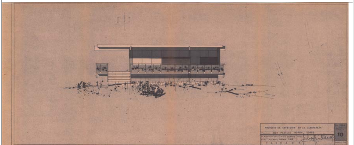
PLANO 10: ALZADO NORTE. E 1/50
